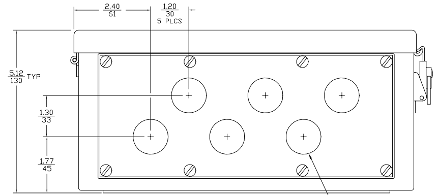
3/4" [19] CONDUIT PLATE Ø.110 / Ø.28 / 6 PLCS
