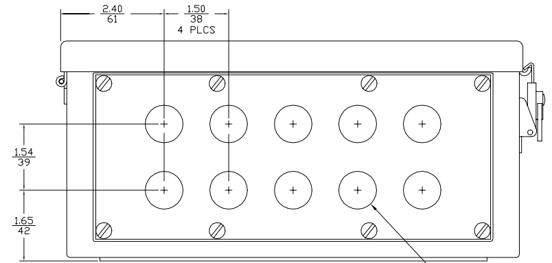
1/2" [13] CONDUIT PLATE Ø.88 / Ø.22 / 10 PLCS
